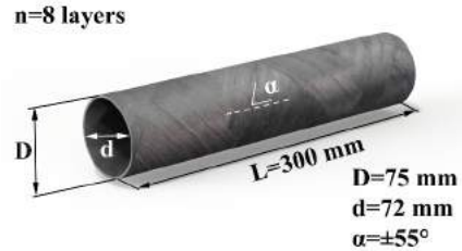
Şekil 1. Kompozit Tüp
