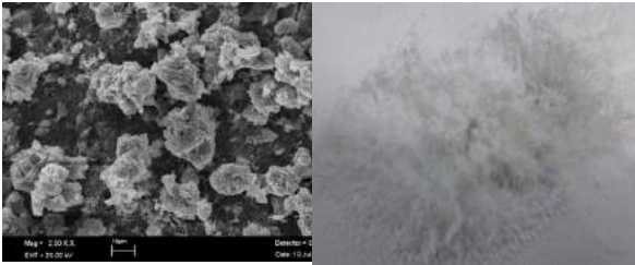
Şekli 3. 17 kV voltaj, 8 cm toplayıcı-iğne ucu mesafesi, 4 ml/saat çözelti besleme hızı, pH 5 değerinde 300 dakikada üretilmiş 3D nanoliflerin SEM ve Kamera görüntüleri (Maleik)
