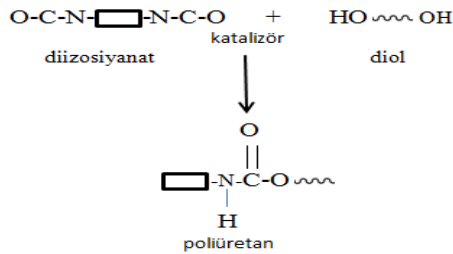
Şekil 1. Poliüretan sentezi
