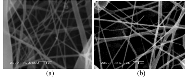
Şekil 1. PLA nanofiberlerin SEM görüntüleri; (a) PLA, (b) PLA/SH.
