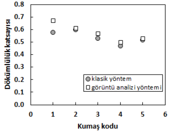
Şekil 5. Dökümlülük katsayısı ölçüm sonuçları
