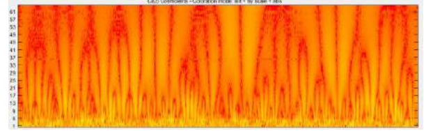
Şekil 7. Skalogram
