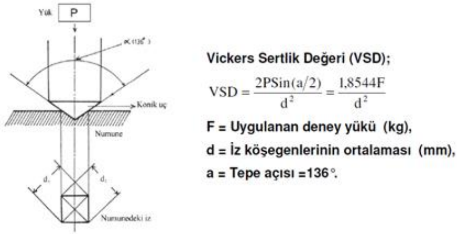
Şekil 3: Vickers Sertlik Deneyi
