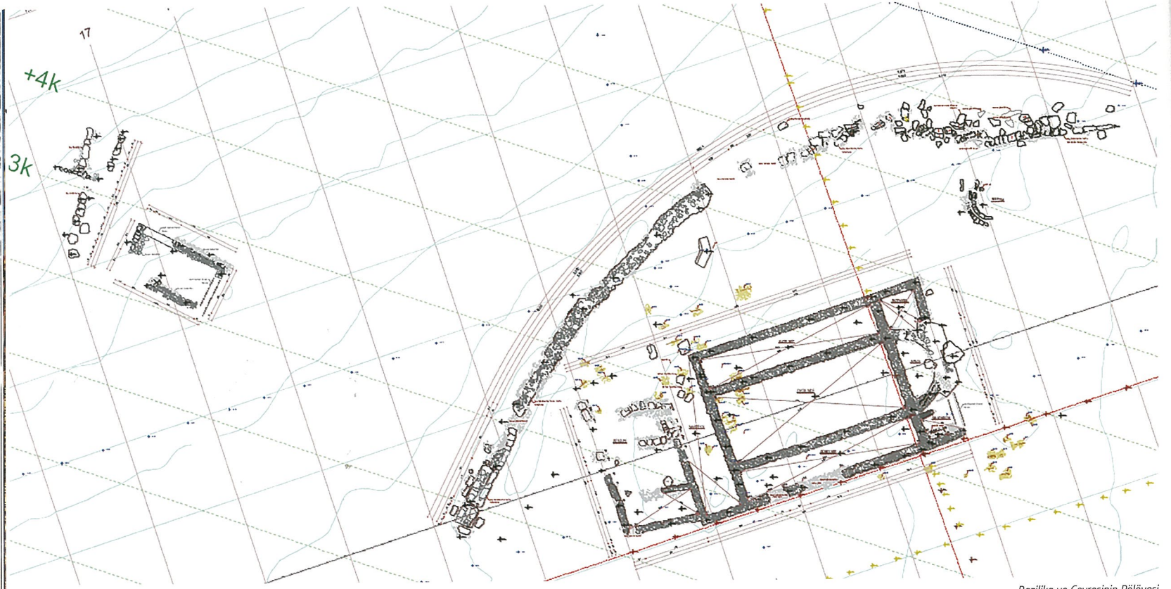
Bazilika ve Çevresinin Rölövesi
